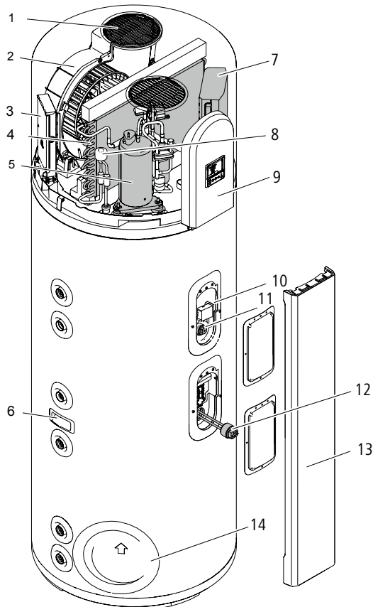
Abb. 1: Komponenten
