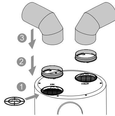
Abb. 11: Typische Installationsarten
