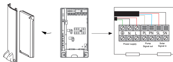
Abb. 9: Netzanschluss
